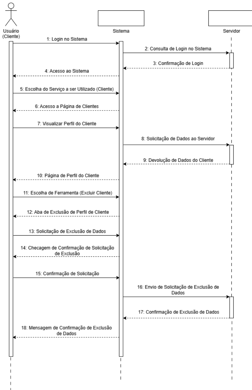
Figura 13 - Diagrama de Sequência: Exclusão de dados
